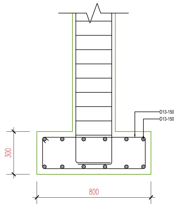
POTONGAN A
